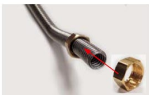
Raccords écrou tournant IR
